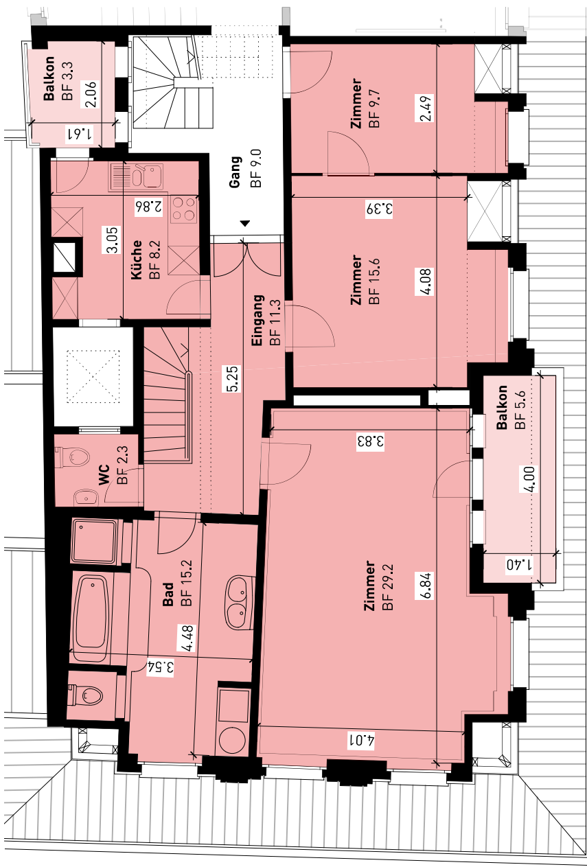
Grundriss 5. Obergeschoss
