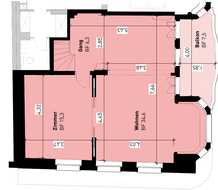
Grundriss 4. Obergeschoss
